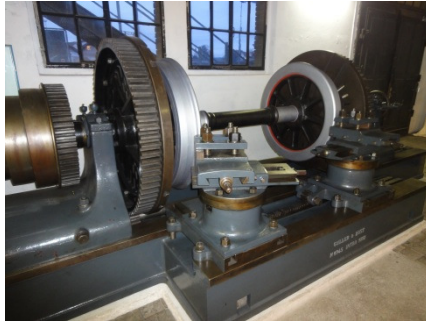
Radsatz Drehbank von 1892
